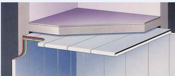
Verstärkung bestehender Massivbau-Tresorräume mit Relastan®-Elementen
